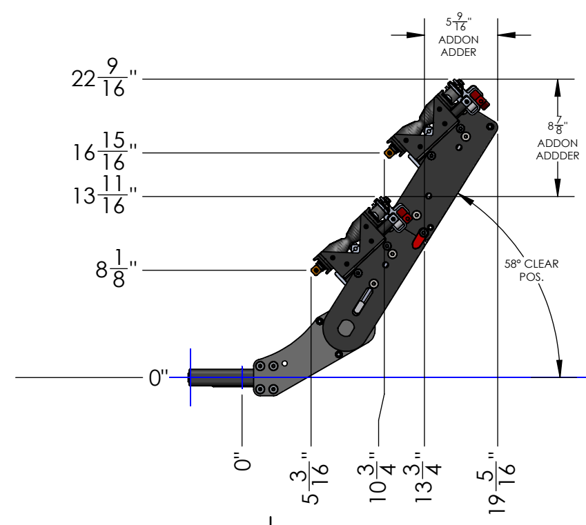
DETAIL 1.25"-REC SCALE 1 : 5
